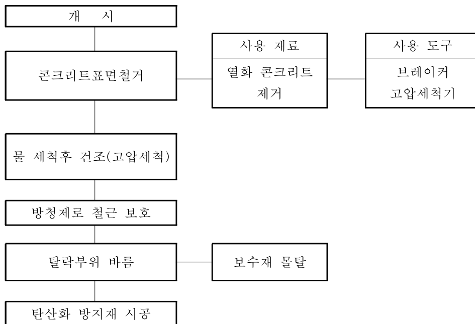
[단면복구공법 시공순서도]
