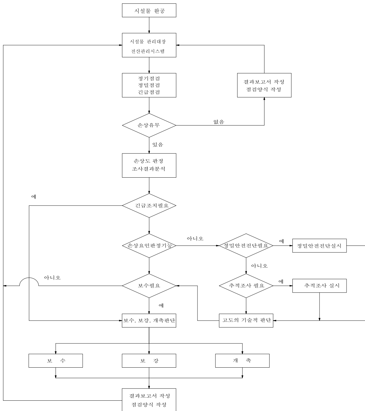
[유지관리 흐름도]
